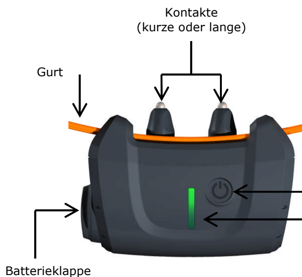
Abb. 1 Das Empfänger-Halsband CANICOM 5
